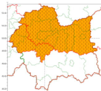
Intensywne opady śniegu 2021-02-07 19:26
